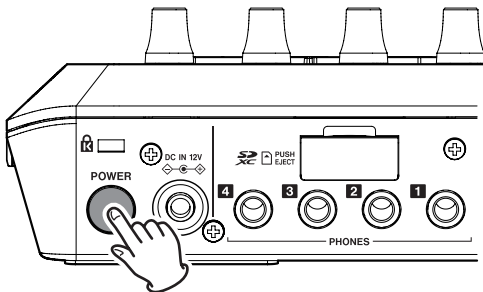
Botón POWER (19)
