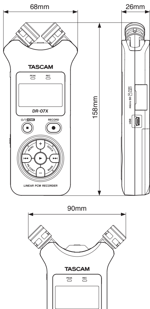
Размеры с раскрытыми микрофонами
