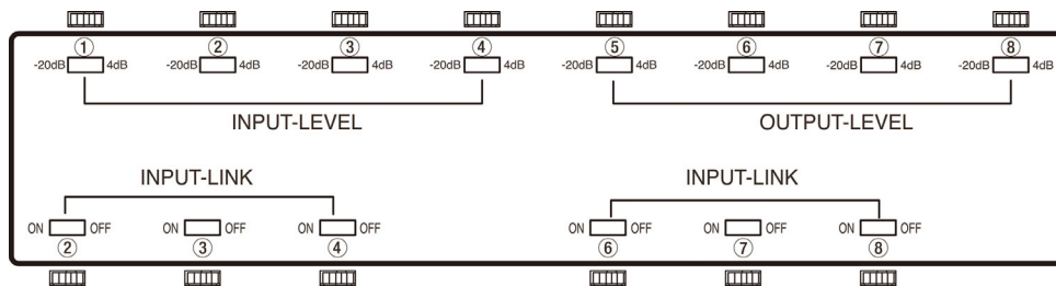
ボトムパネル (INPUT LEVEL、OUTPUT LEVEL、INPUT LINK スイッチ)
