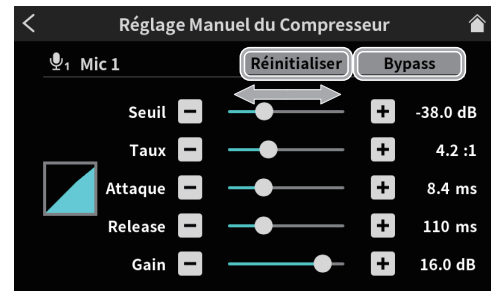
Écran Réglage manuel du compresseur
