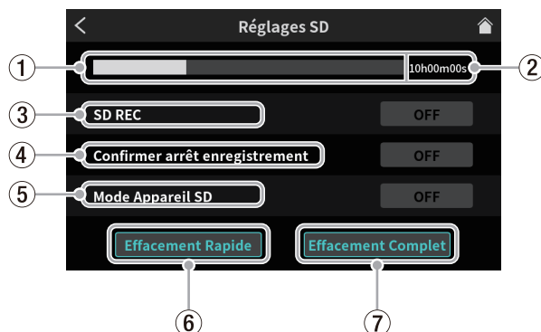
Écran Réglages SD
